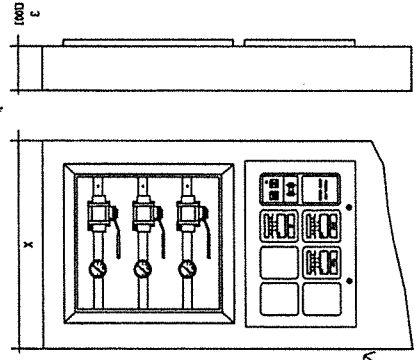
DETAIL การติดตั้ง ZONE VALVE IN BOX w/GAUGE & ALARM ติดตั้งจากตู้ควบคุมบริเวณ 1.30 ชั้น 7
